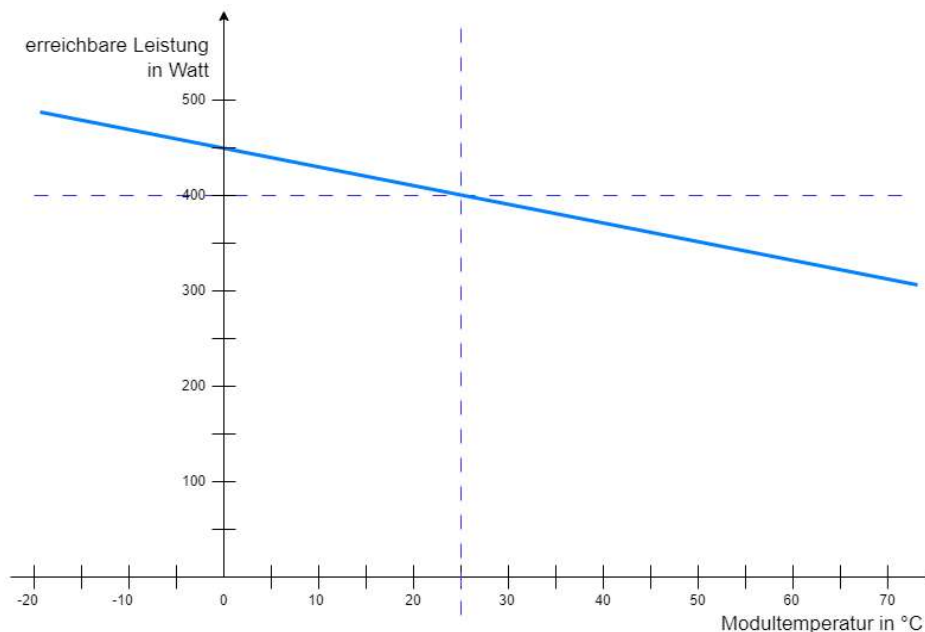
Temperatur-Abhängigkeit am Beispiel eines Solarmoduls mit 400 Wp
